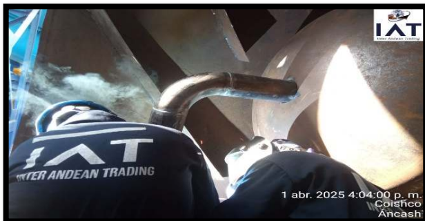
SOLDEO DE TUBERIA DE VAPOR
